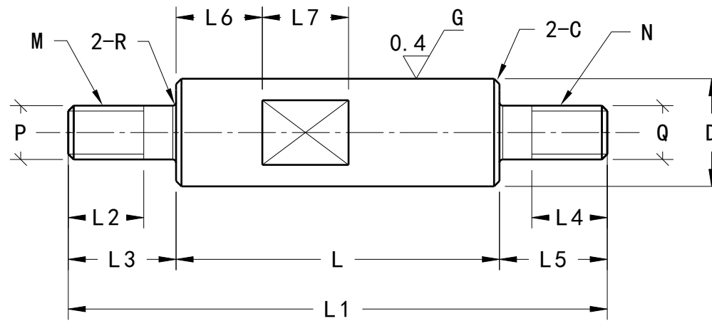
右視圖 縮放: 2:1
