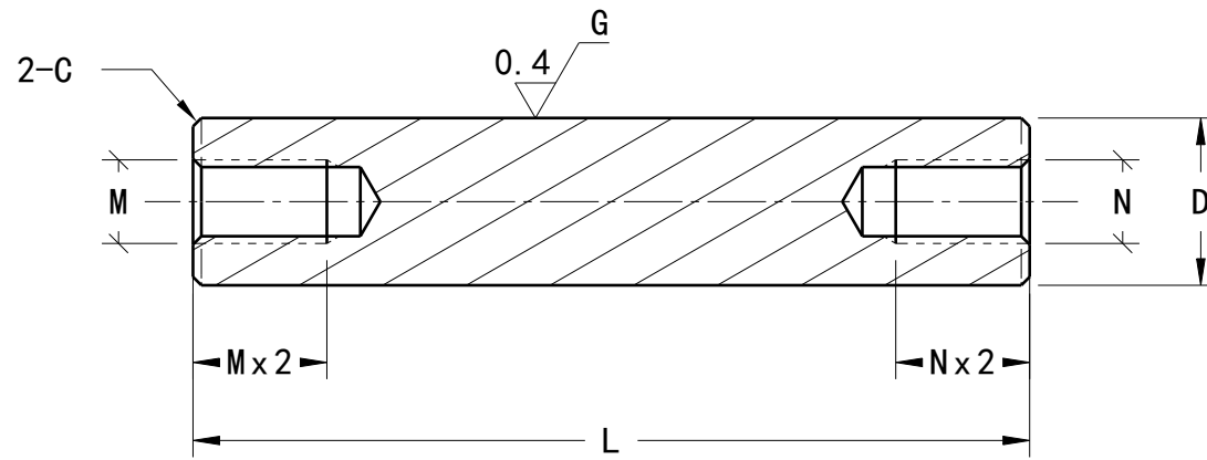
Section view A-A Scale: 2:1
