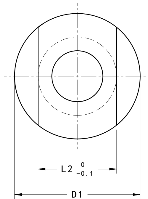
右視圖 縮放: 7:2
