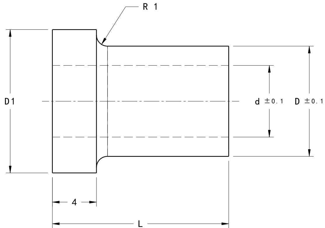
前視圖 縮放： 5:1
