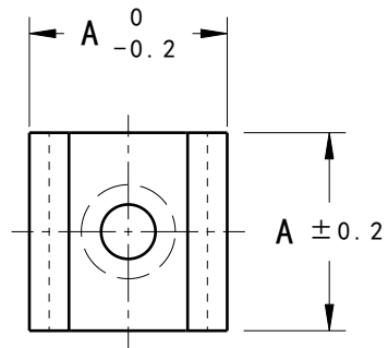
前視圖 縮放: 6:5
