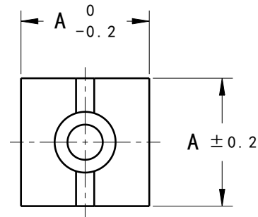
前視圖 縮放: 6:5
