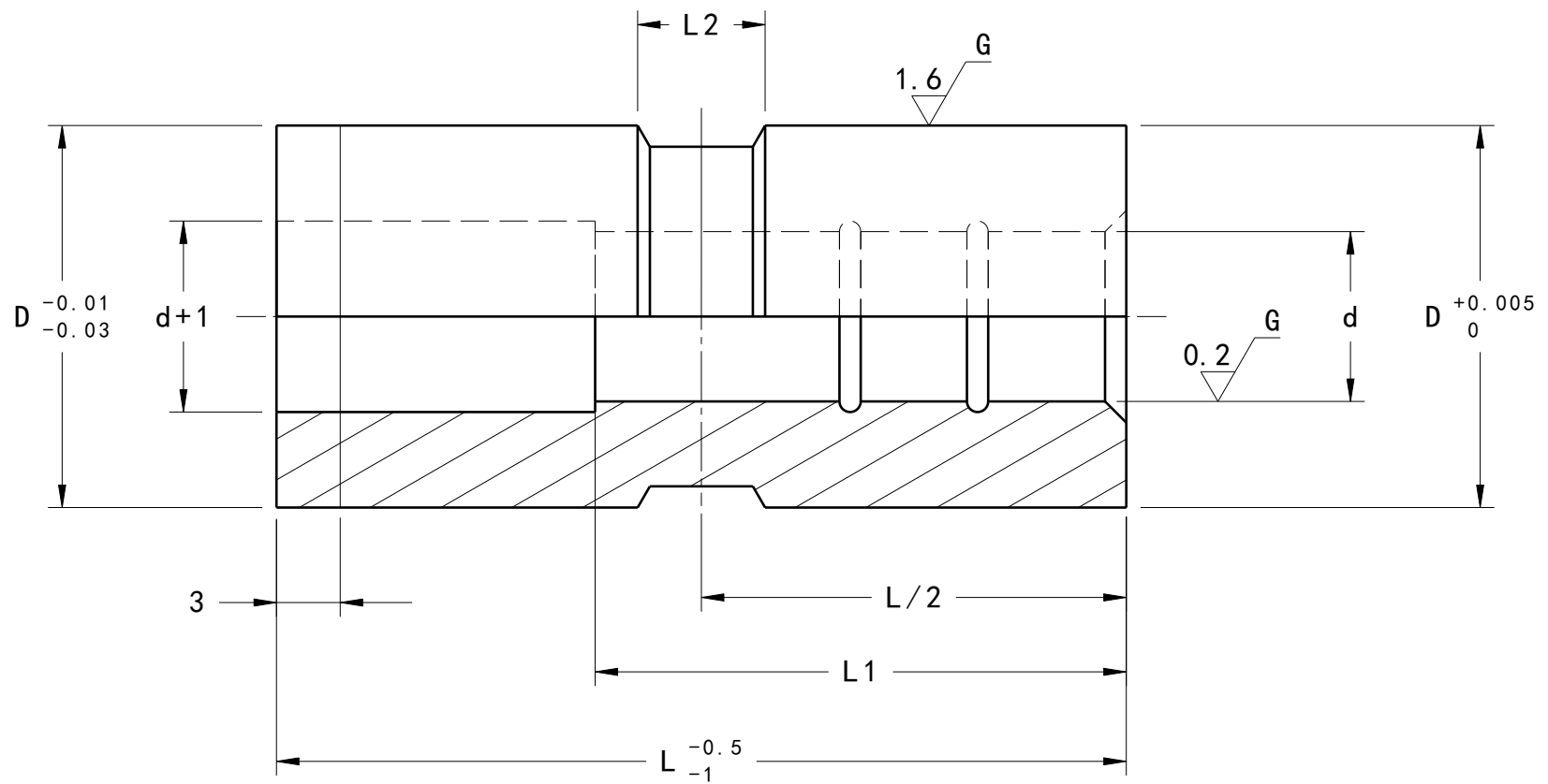
剖面視圖A-A 縮放: 3:1
